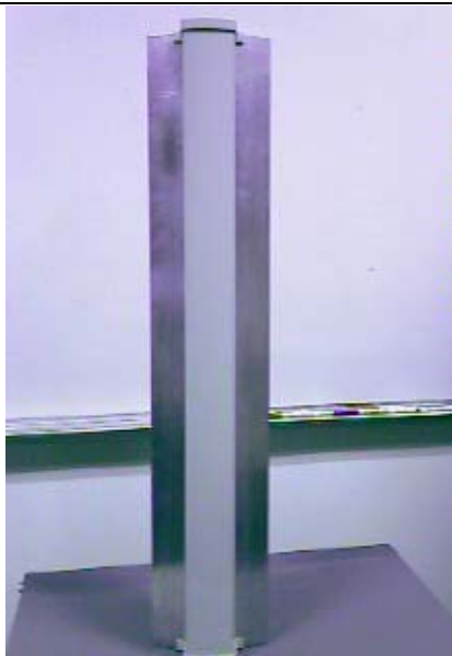
Figura 3.5 Antena sectorial de 14.5 dBi. Vista frontal
