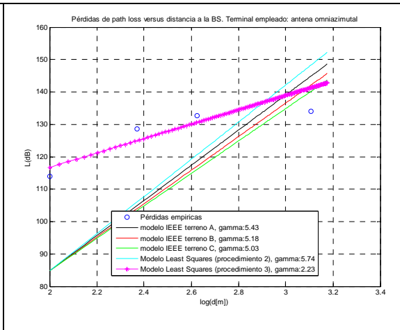
Figura 4.20 Pérdidas empíricas y modelos distintos de path loss versus distancia. Terminal empleado: antena omni-azimutal
