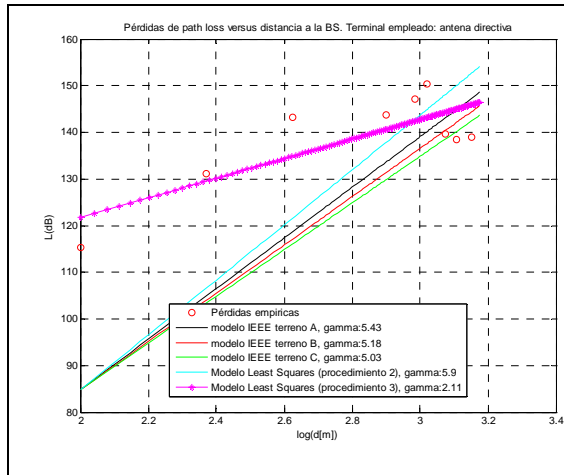
Figura 4.19 Pérdidas empíricas y modelos distintos de path loss versus distancia. Terminal empleado: antena direccional
