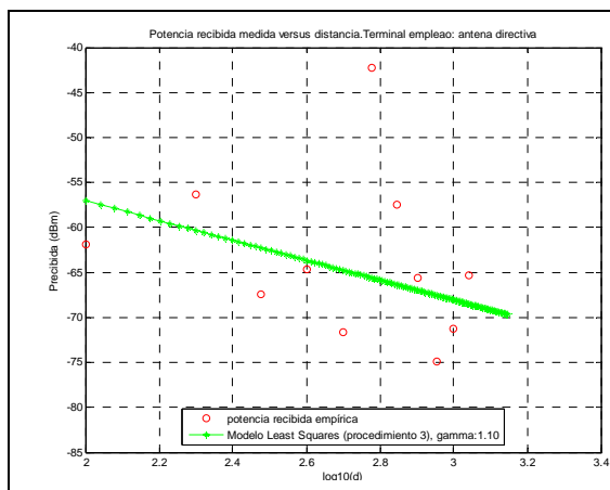
Figura 4.31 Potencia recibida empírica y modelo empírico versus distancia a la BS. Terminal empleado: Antena directiva
